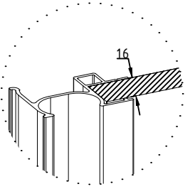
Panneau : épaisseur 16mm
