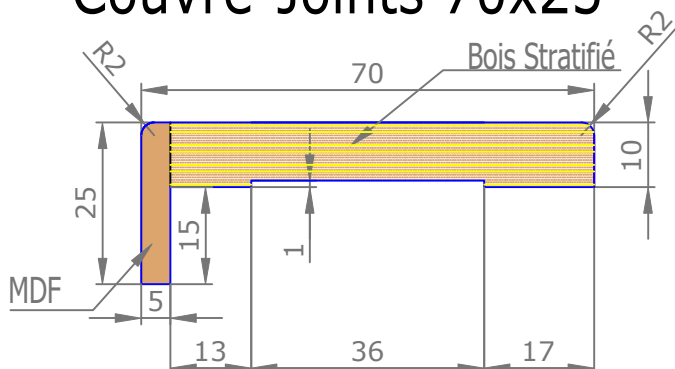
Couvre-Joints 70x25
