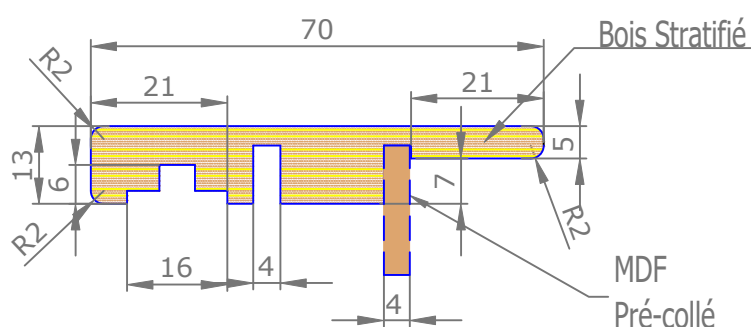
Couvre-Joints 70x13
