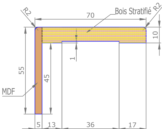
Couvre-Joints 70x55
